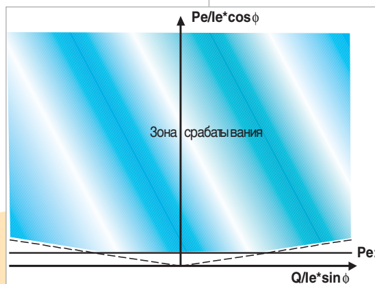
Ваттметрическая хар-ка
