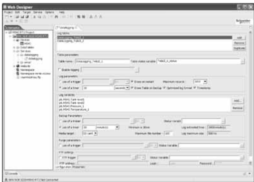
Конфигурирование функции регистратора данных Data Logging для модуля BMX NOR 0200H
