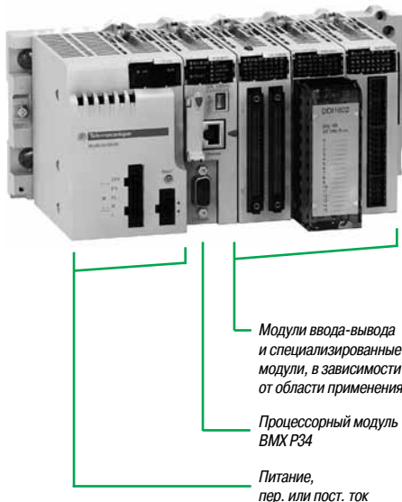
Платформа автоматизации Modicon M340
