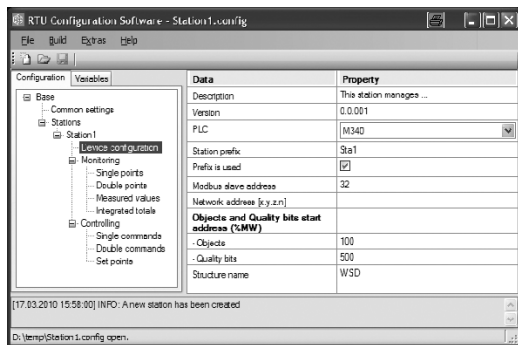
Экран конфигурации RTU
