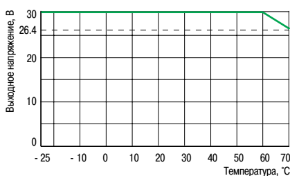
BMX DDM 16022H, транзисторные выходы
