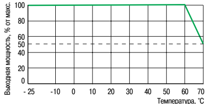
BMX DDM 16025H, релейные выходы 24 В пост. или 240 В пер. тока
