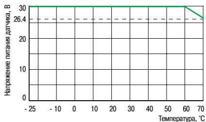
BMX DDM 16025H, входы 24 В пост. тока
