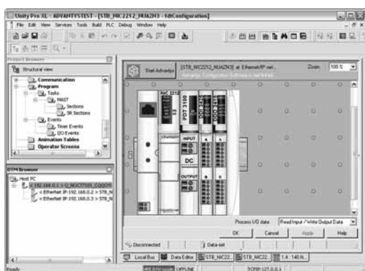
Редактор DTM (узел Modicon STB)
