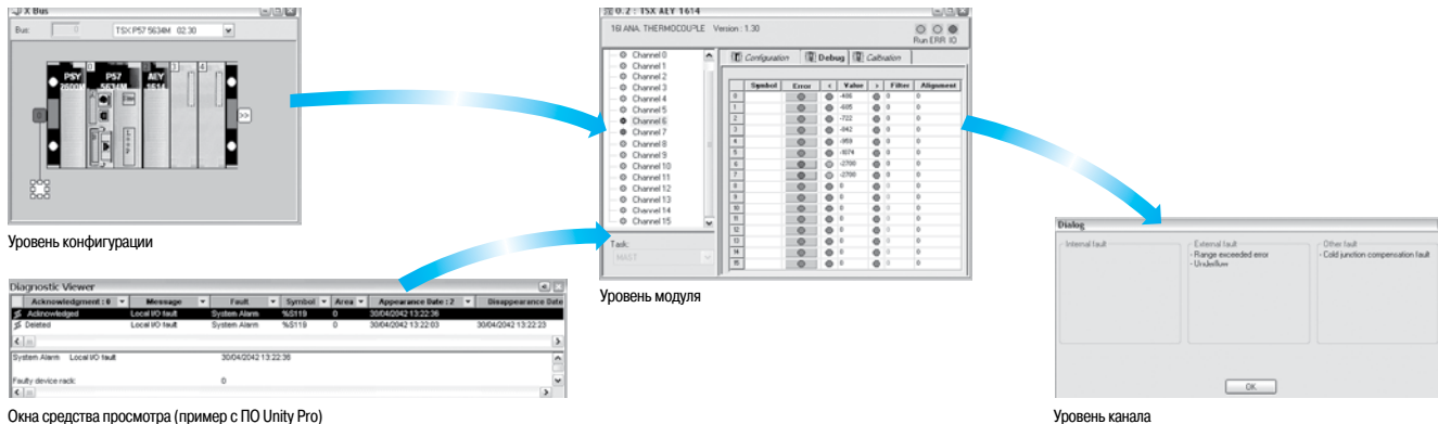
Окна средства просмотра (пример с ПО Unity Pro)
