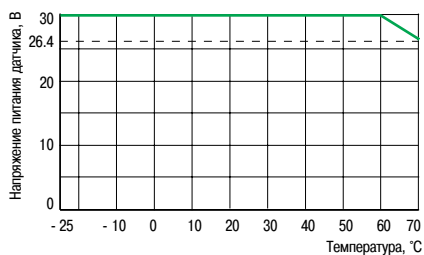
BMX DDM 16022H, входы 24 В пост. тока
