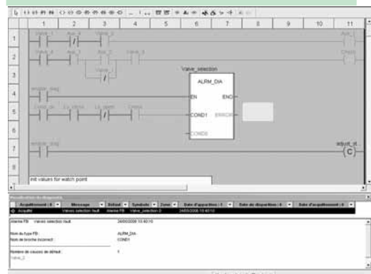
Диагностика с анализом причины сбоя
