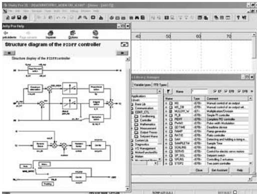
CONT_STL, встроенное в Unity Pro программирование управления производственным процессом
