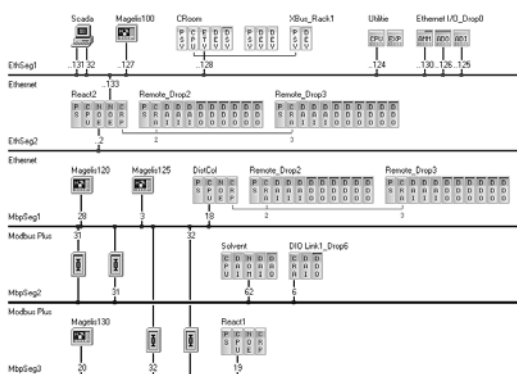
Конфигурация системы автоматизации с несколькими станциями
